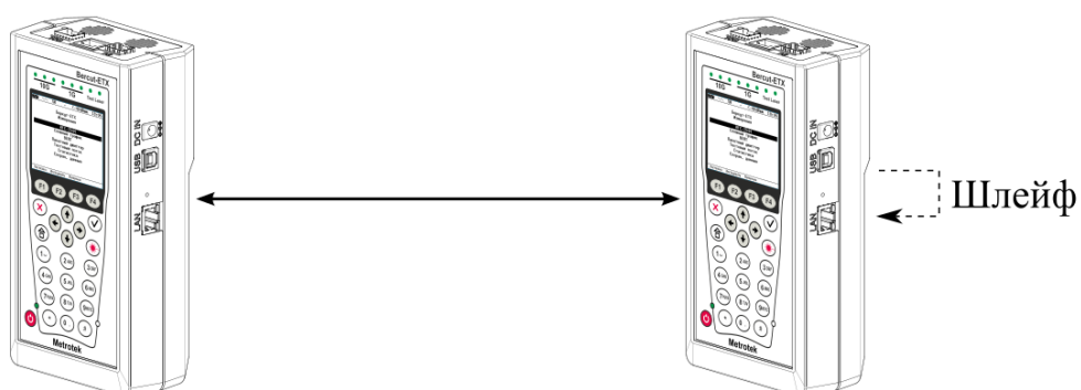
Рисунок 19.8. Тестирование на физическом уровне (вариант 1)
