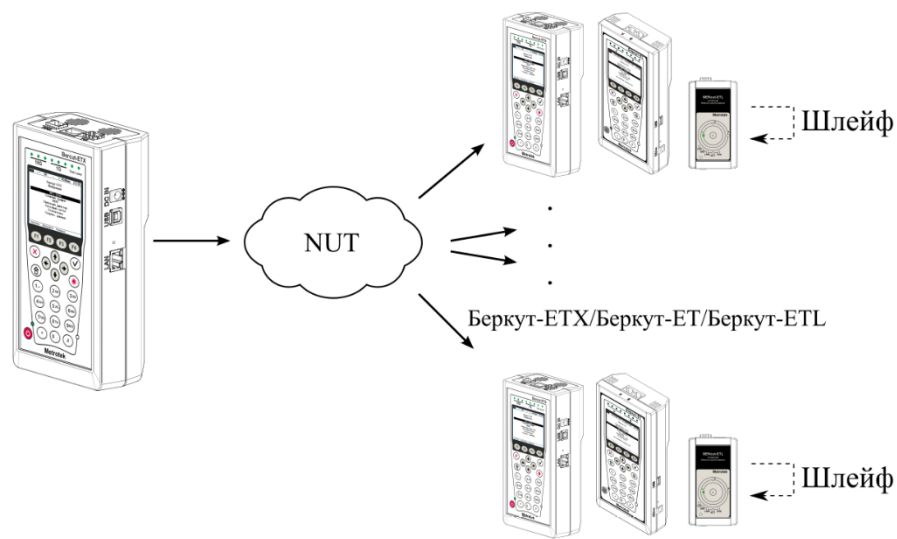
Рисунок 16.1. Схема тестирования
