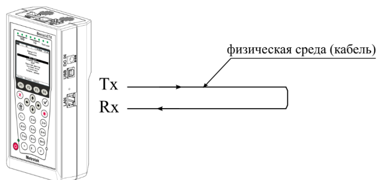
Рисунок 19.8. Тестирование на физическом уровне (вариант 1)
