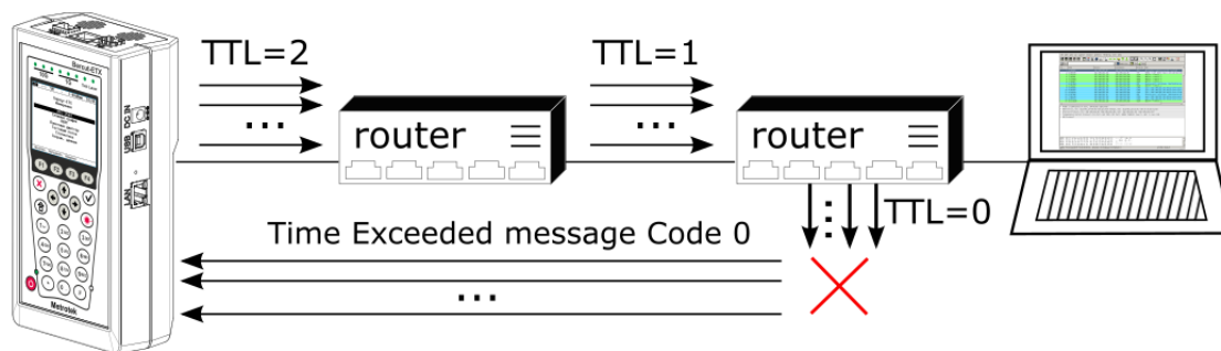
Рисунок 21.5. Проверка устойчивости маршрутизатора к приёму пакетов с TTL=0
