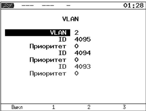
Рисунок 9.5. Меню «VLAN»
