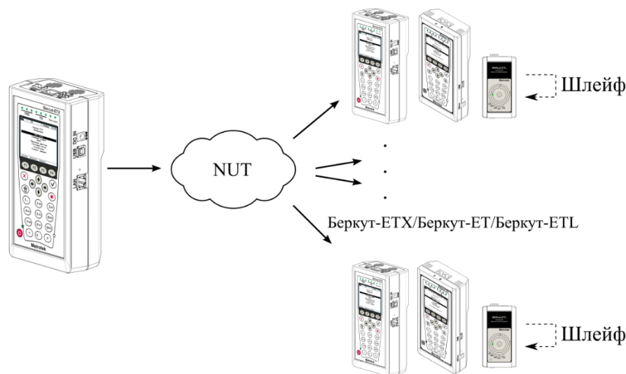
Рисунок 16.1. Схема тестирования
