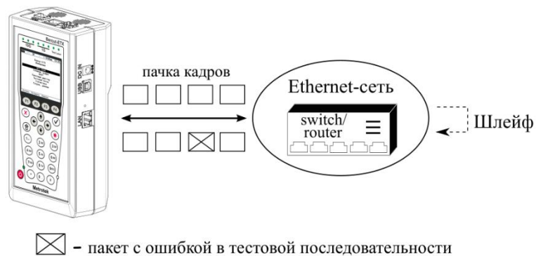
Рисунок 19.11. Тестирование на канальном/сетевом уровне (вариант 2)
