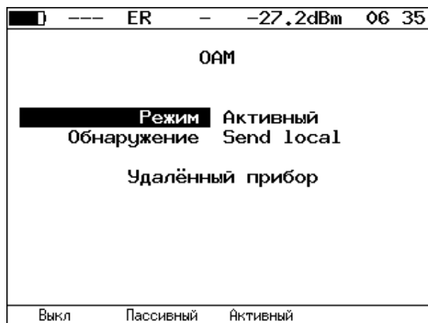
Рисунок 15.2. Меню «OAM»
