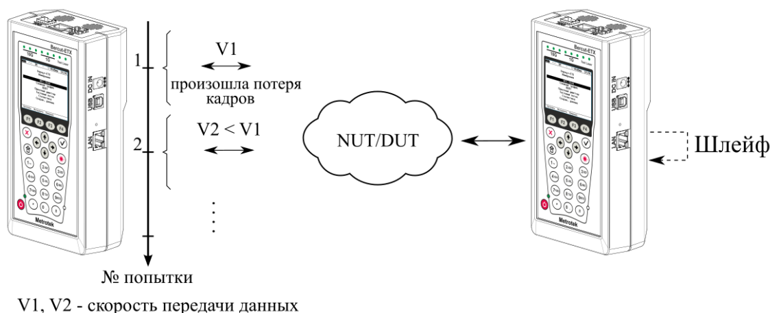
Рисунок 8.1. Анализ пропускной способности
