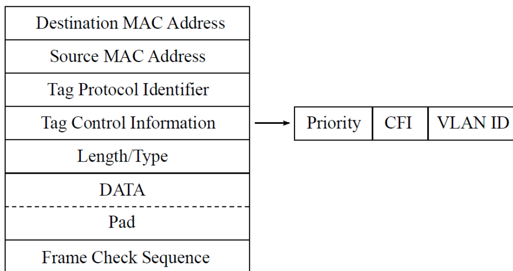
Рисунок 34.2. Структура Ethernet-кадра, содержащего VLAN-метку
