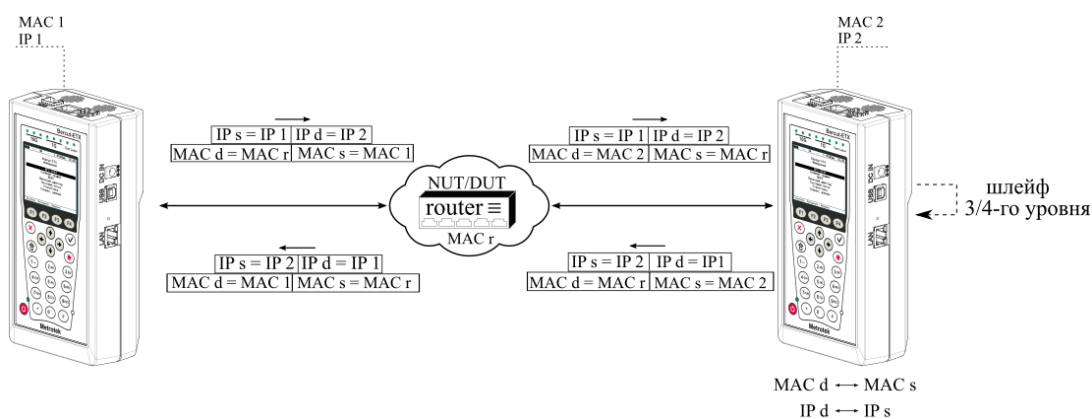
Рисунок 6.2. Типовая схема подключения 2
