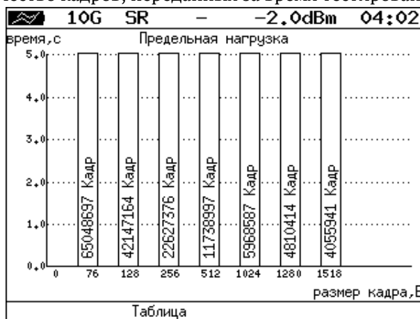
Рисунок 10.8. Результаты теста: график
