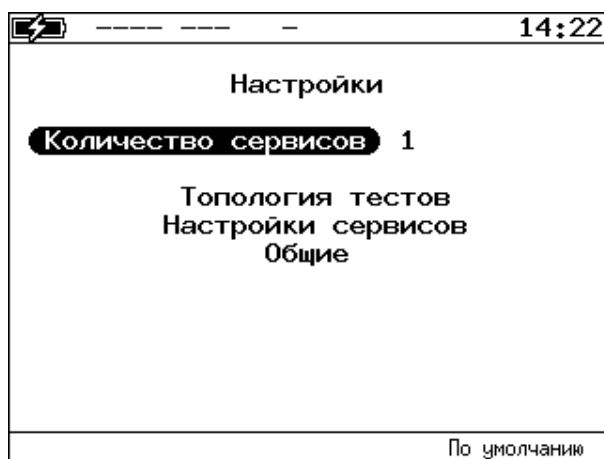
Рисунок 12.2. Меню «Настройки»
