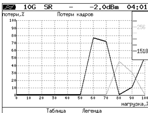
Рисунок 10.6. Результаты теста: график
