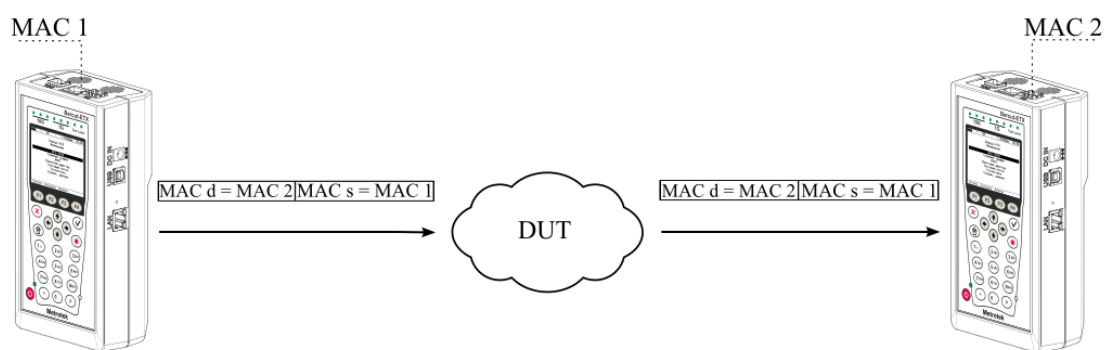
Рисунок 6.3. Типовая схема подключения 3
