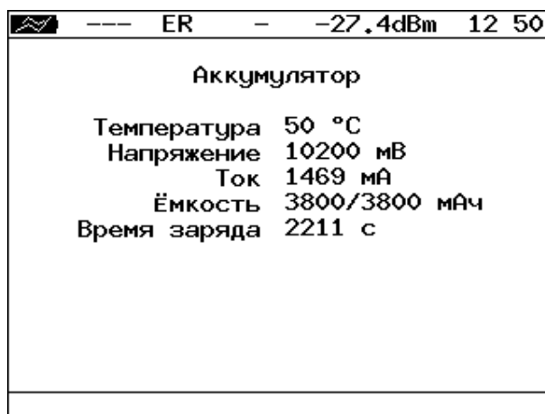
Рисунок 26.7. Экран «Аккумулятор»
