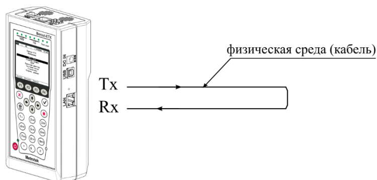
Рисунок 19.8. Тестирование на физическом уровне (вариант 1)
