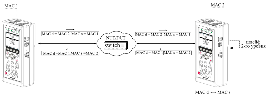
Рисунок 6.1. Типовая схема подключения 1
