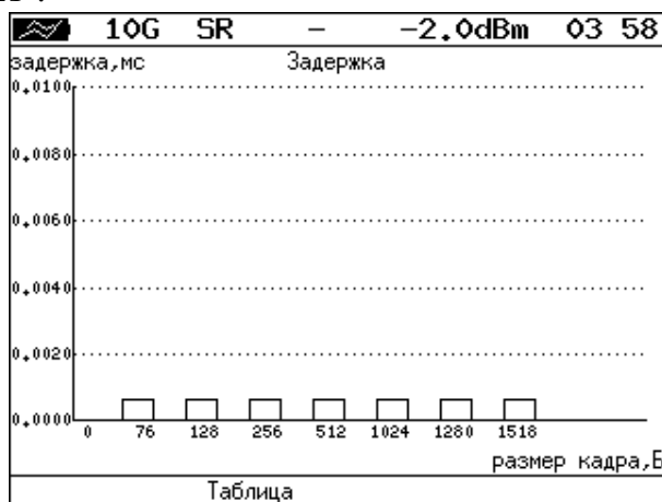
Рисунок 10.4. Результаты теста: график
