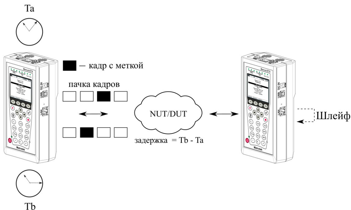
Рисунок 8.2. Анализ задержки
