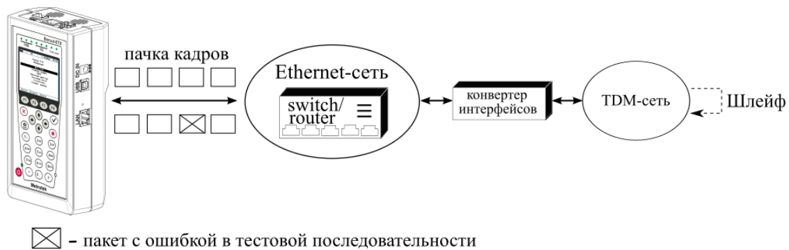
Рисунок 19.10. Тестирование на канальном/сетевом уровне (вариант 1)
