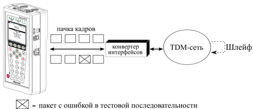
Рисунок 19.12. Тестирование на канальном/сетевом уровне (вариант 3)
