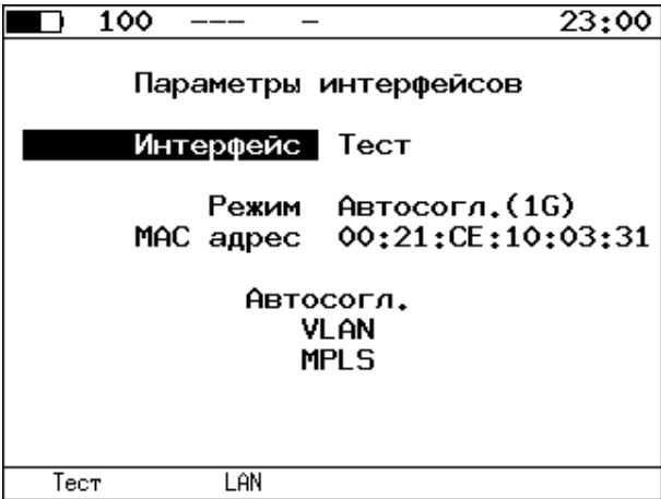
Рисунок 27.1. Меню «Параметры интерфейсов»
