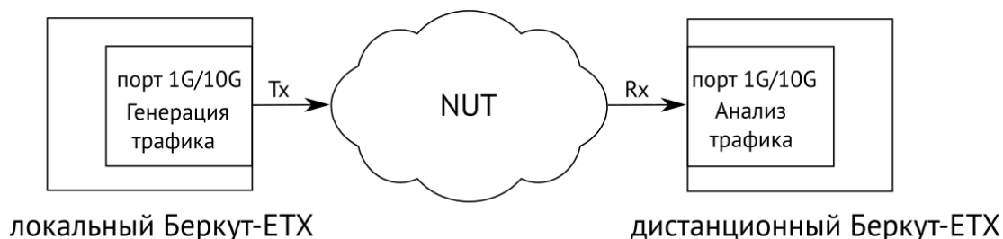
Рисунок 8.1. Схема однонаправленного теста
