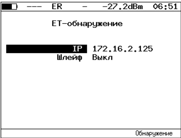
Рисунок 17.2. Меню «ЕТ-обнаружение»
