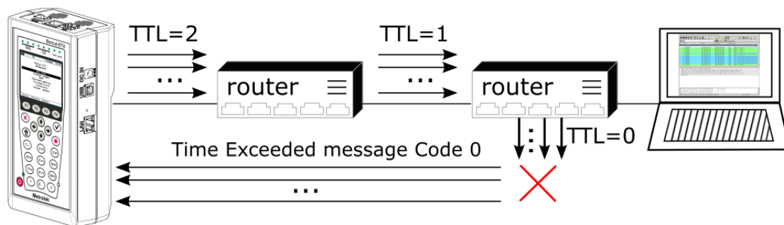
Рисунок 22.5. Проверка устойчивости маршрутизатора к приёму пакетов с TTL=0
