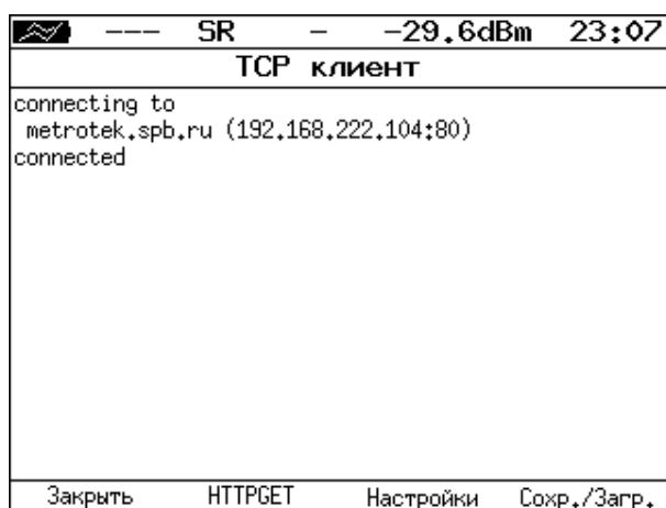
Рисунок 18.14. Пример успешного соединения с узлом
