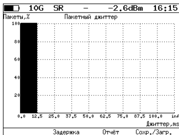
Рисунок 21.3. Экран «Пакетный джиттер» (график)
