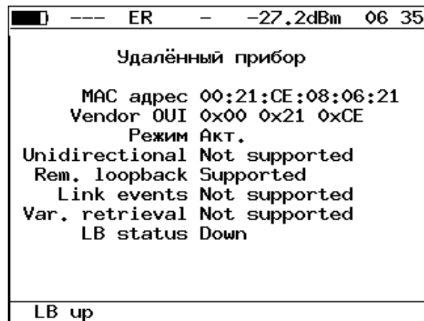
Рисунок 16.3. Меню «Удалённый прибор»
