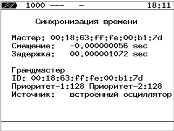
Рисунок 28.4. Информация о синхронизации времени
