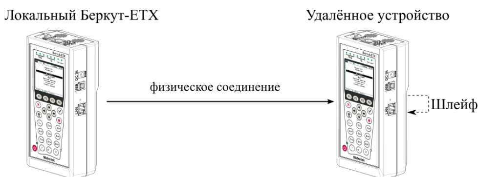
Рисунок 16.1. Схема тестирования
