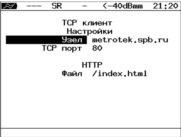
Рисунок 18.13. Настройки теста «TCP клиент»
