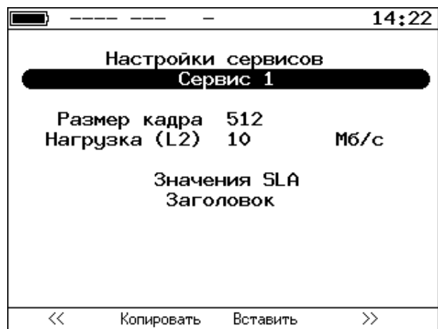
Рисунок 13.4. Меню «Настройки сервисов»
