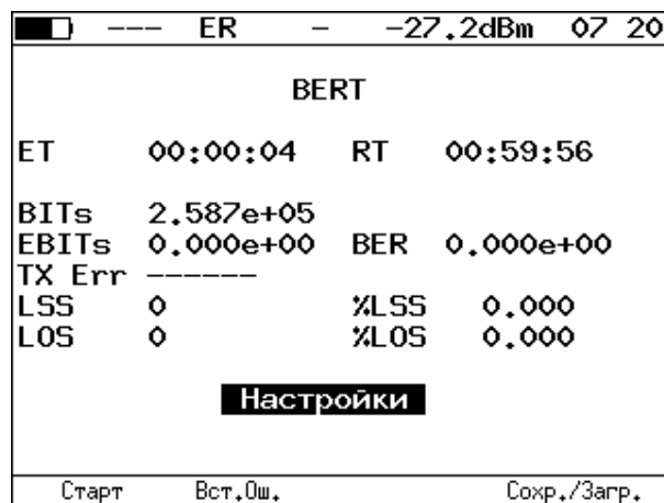
Рисунок 20.5. Экран «BERT»
