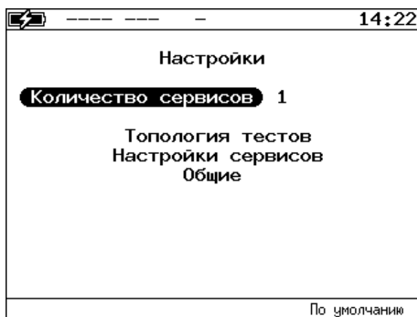
Рисунок 13.2. Меню «Настройки»
