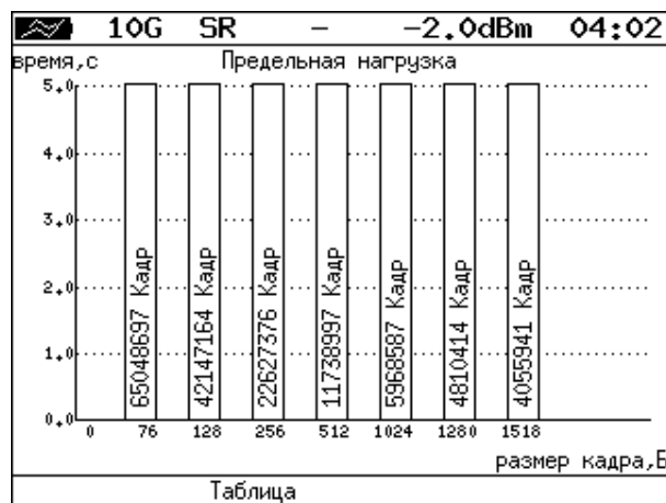
Рисунок 11.8. Результаты теста: график
