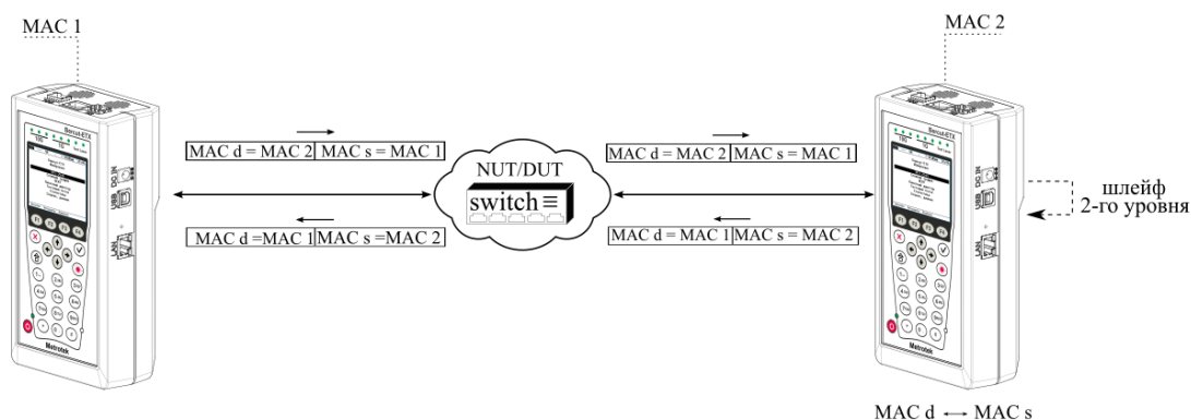
Рисунок 7.1. Типовая схема подключения 1
