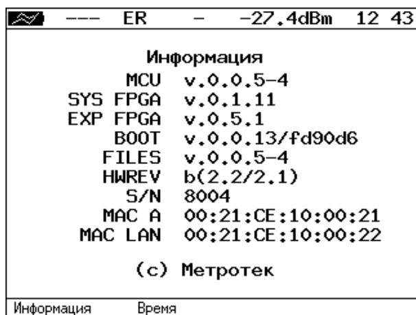
Рисунок 28.5. Экран «Информация»
