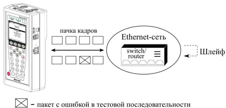
Рисунок 20.11. Тестирование на канальном/сетевом уровне (вариант 2)
