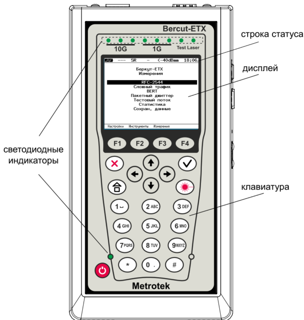
Рисунок 5.1. Лицевая панель
