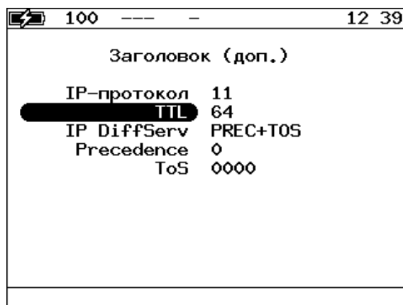
Рисунок 10.3. Настройка IP
