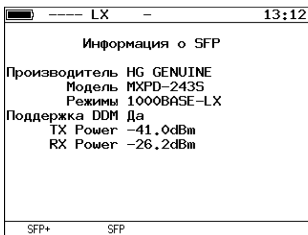
Рисунок 28.6. Экран «Информация о SFP»
