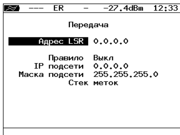
Рисунок 27.4. Меню «Передача»
