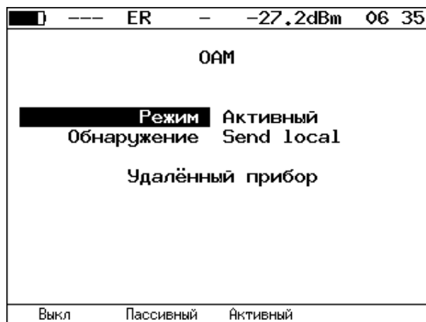
Рисунок 16.2. Меню «OAM»
