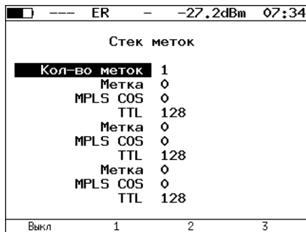
Рисунок 20.7. Меню «MPLS»
