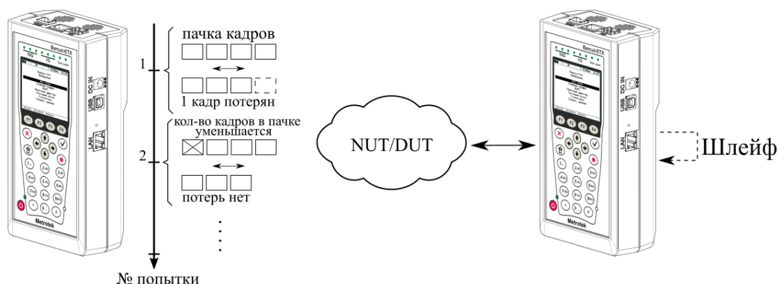
Рисунок 9.4. Анализ предельной нагрузки
