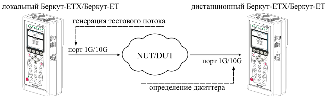
Рисунок 22.3. Генерация постоянного трафика. Схема 2
