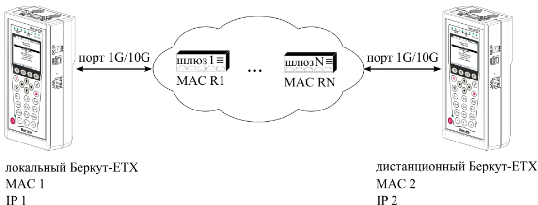
Рисунок 8.2. Типовая схема подключения
