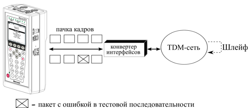
Рисунок 20.12. Тестирование на канальном/сетевом уровне (вариант 3)
