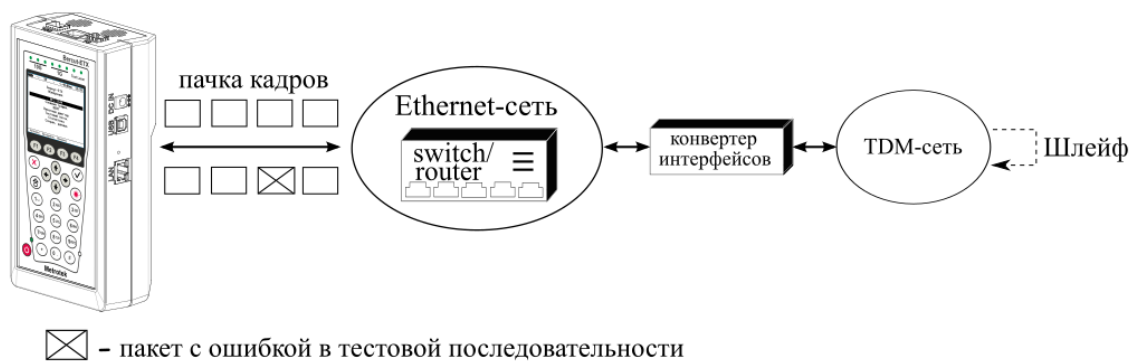
Рисунок 20.10. Тестирование на канальном/сетевом уровне (вариант 1)
