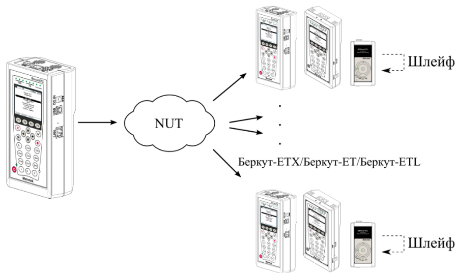
Рисунок 17.1. Схема тестирования
