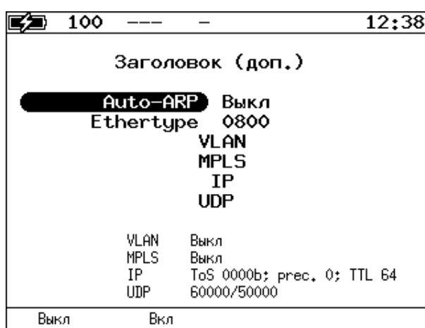
Рисунок 10.2. Меню «Заголовок (доп.)»
