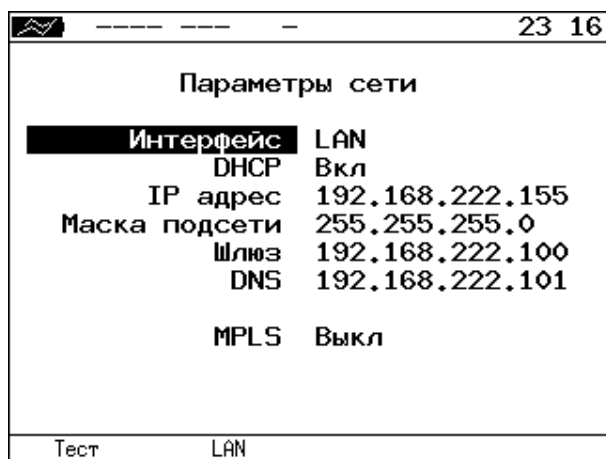
Рисунок 26.1. Меню «Параметры сети»
