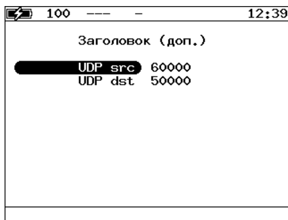
Рисунок 10.4. Настройка UDP
