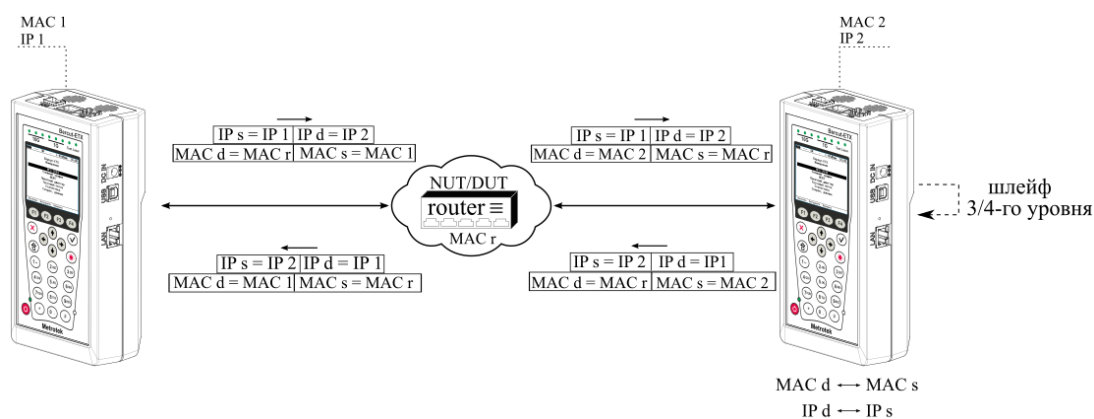
Рисунок 7.2. Типовая схема подключения 2
