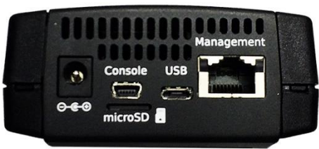
Рисунок 3.4. Задняя панель варианта исполнения M716-02-001/2
