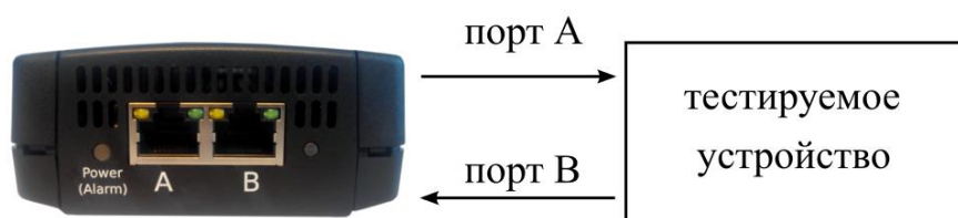
Рисунок 21.1. Типовая схема подключения для проведения теста «Тестовые данные»
