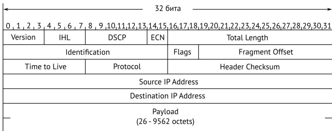
Рисунок 23.3. Структура пакета 3-го уровня
