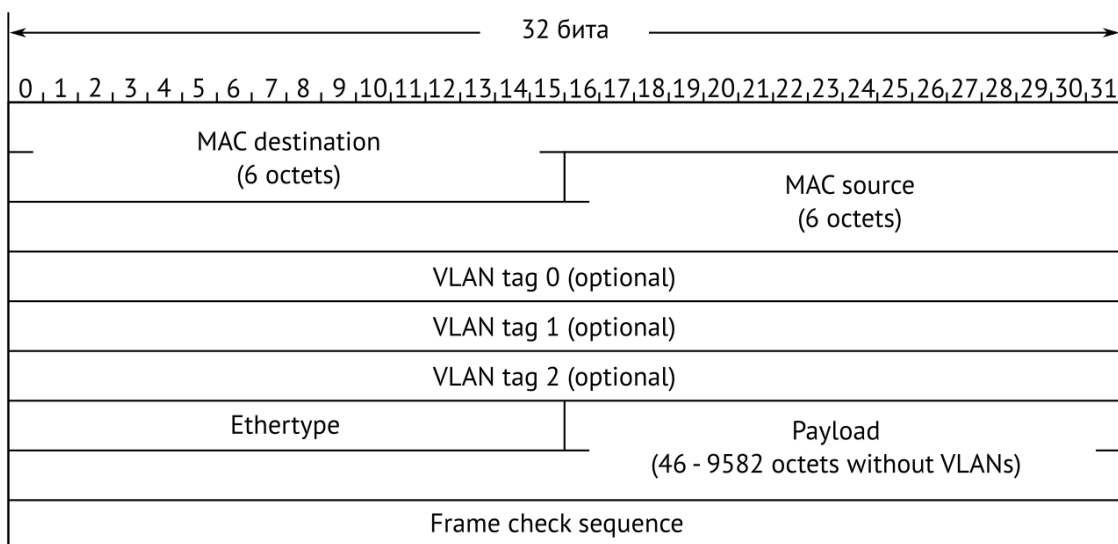
Рисунок 23.2. Структура кадра 2-го уровня
