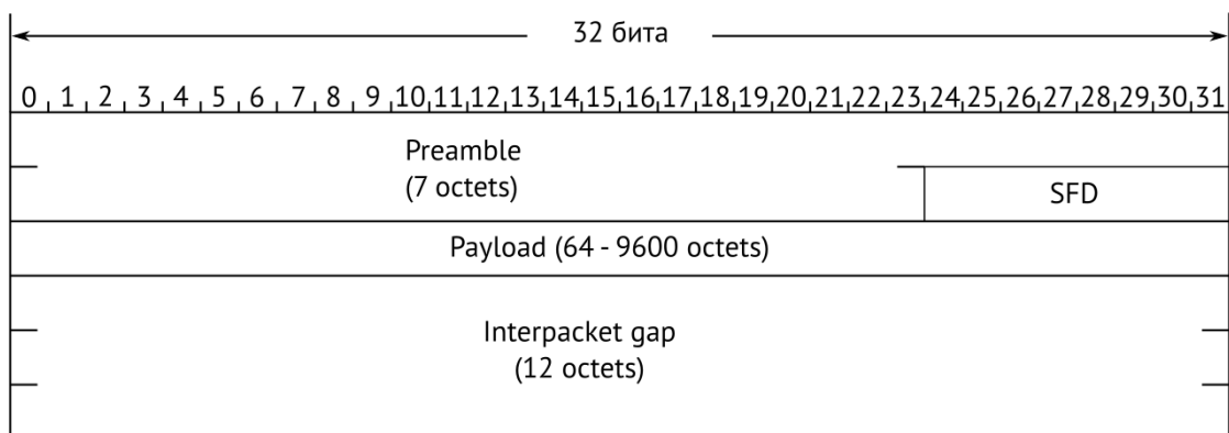
Рисунок 23.1. Структура пакета 1-го уровня
