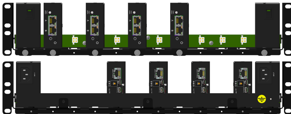
Рисунок 7.1. Установка приборов в полку-шасси
